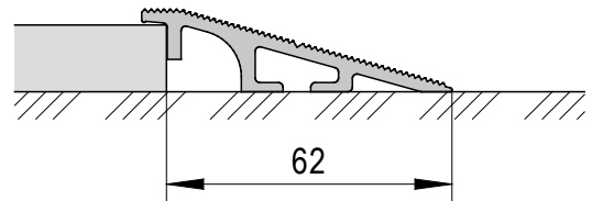
Rampenschiene RS 14
