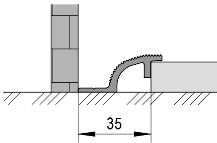
Befestigungsschiene BS 14
