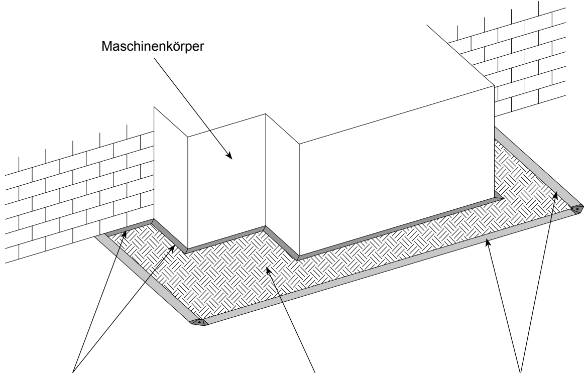
Befestigungsschiene BS 14 im Wand- und Maschinenbereich
